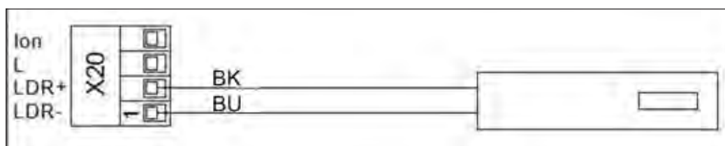
Рис. 11-11 Фото Сопротивление подключения, например Siemens QRB...
