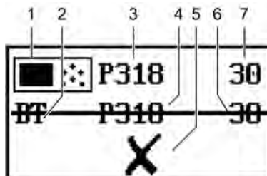
Рис. 5-29 Дисплей неправильной передачи данных
