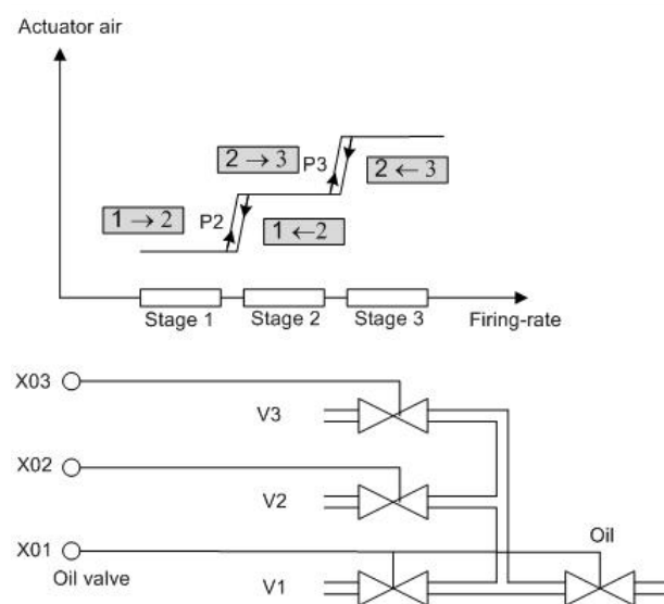
Рис. 5-39 3-этапное функционирование
