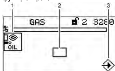
Рис. 5-35 Меню растопочной горелки при масляном функционировании
