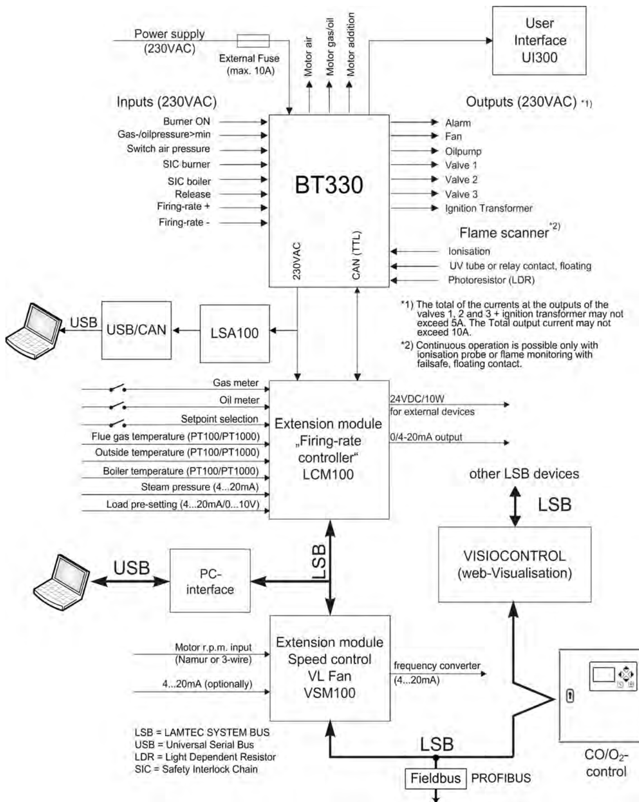
Рис. 11-1 Осмотр системы BurnerTronic BT300
