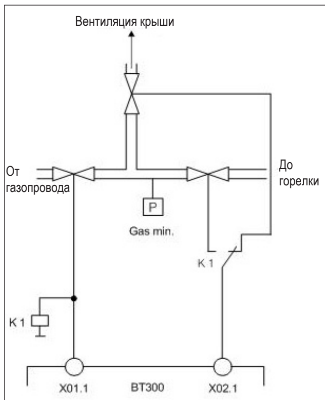
Рис. 8-2 Предложение для прокладки электрических проводов для вентиляции газовой линии через крышу с BurnerTronic
