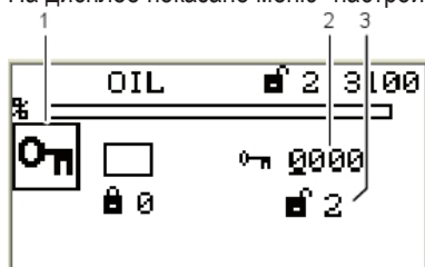
Рис. 5-24 Вводить меню пароля
