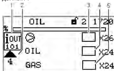
Рис. 5-21 Страница 4 меню цифровых выходных данных
