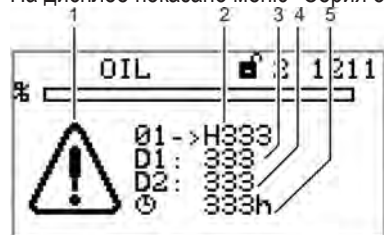
Рис. 5-8 Меню серии ошибок
