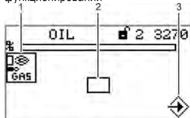
Рис. 5-34 Меню растопочной горелки при газовом функционировании
