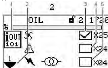
Рис. 5-18 Страница 1 меню цифровых выходных данных
