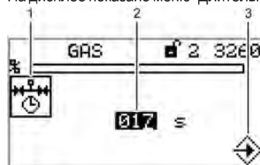
Рис. 5-33 Меню теста утечки клапана.
