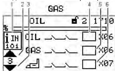
Рис. 5-16 Страница 3 меню входных данных
