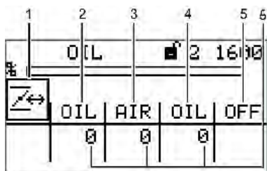
Рис. 5-12 Меню запусков для проведения в действие
