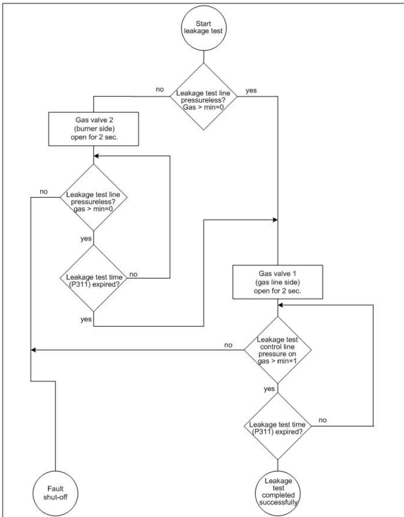
Fig. 8-1 Схема процесса теста утечки
