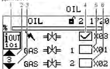
Рис. 5-20 Страница 3 меню цифровых выходных данных
