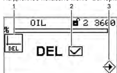
Рис. 5-41 Меню вычеркивания кривых
