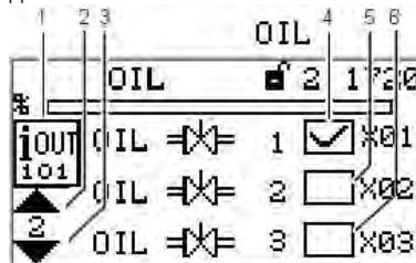
Рис. 5-19 Страница 2 меню цифровых выходных данных
