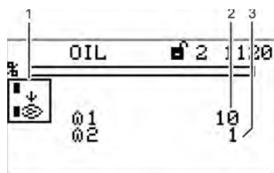
Рис. 5-6 Дисплей "Счетчик пусков"
