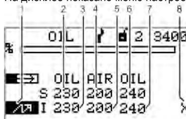
Рис. 5-37 меню настроек кривой
