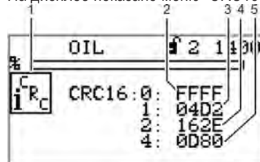
Рис. 5-10 CRC16 меню контрольных сумм
