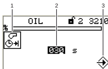
Рис. 5-26 Меню длительности предварительной вентиляции
