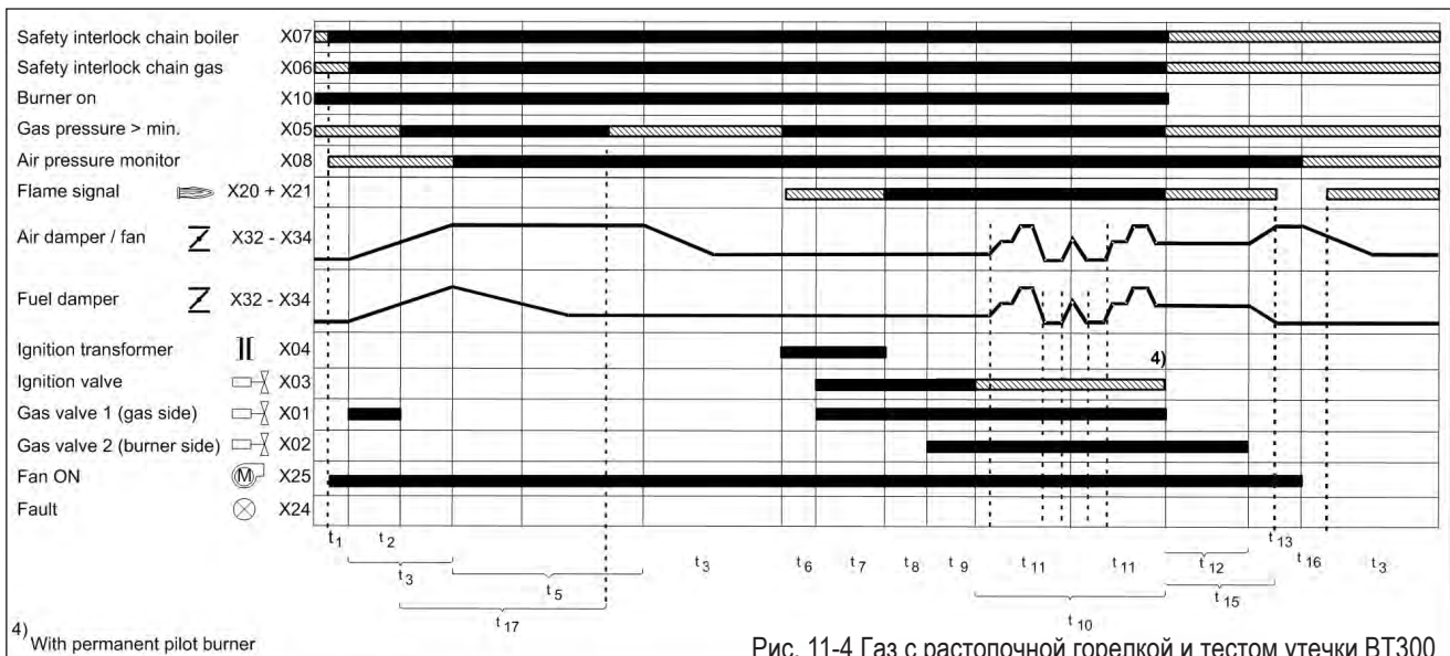
Рис. 11-4 Газ с растопочной горелкой и тестом утечки BT300
