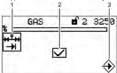
Рис. 5-31 Меню теста утечки клапана перед розжигом.
